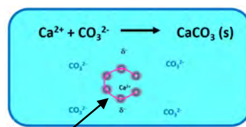
Polyfosfátový řetězec
